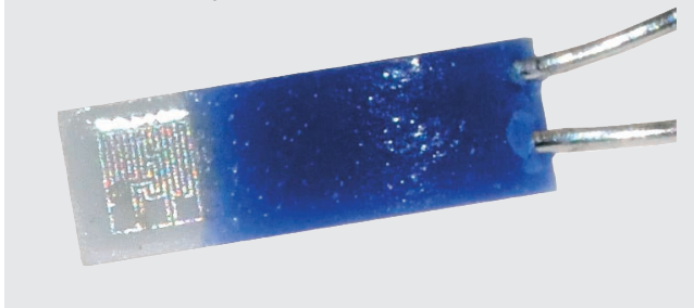
Resistor de medição tipo filme (Thin-film)
