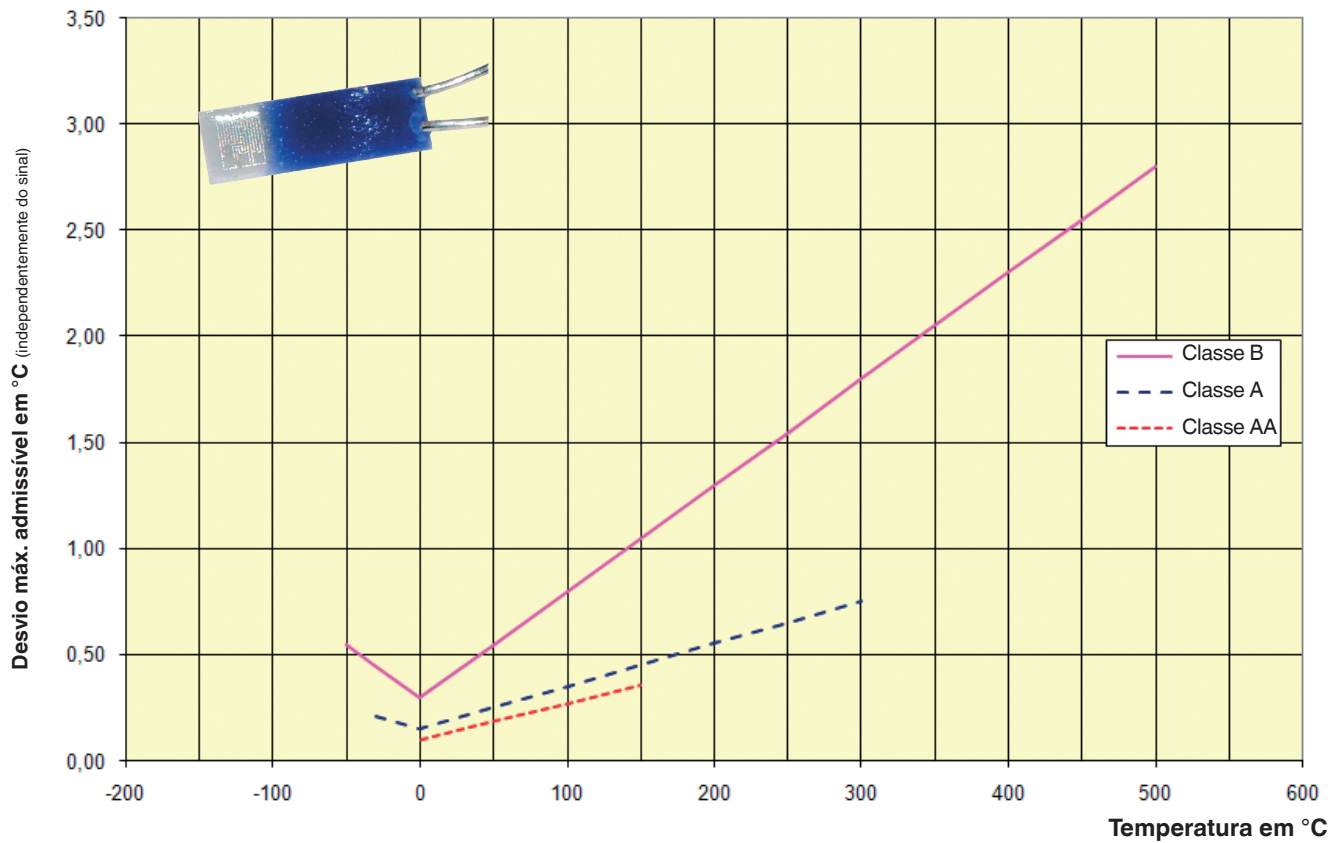
Valor de tolerância IEC 60751: 2008 para termorresistências com resistor de medição tipo fio enrolado
