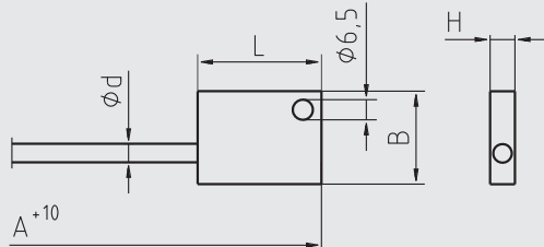
Модель TR50-O, с металлическим контактным блоком со сверленными отверстиями
